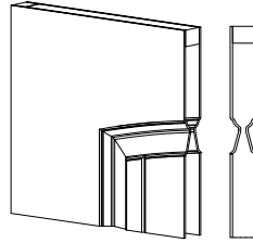
OVOLO STICKING
